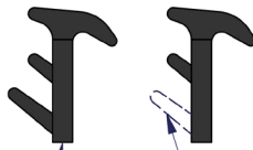
Dichtung 8844KU3 Seal 8844KU3
